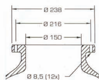
Priključak za tank 6"
