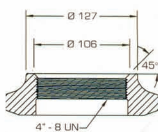
Priključak za tank 4"
